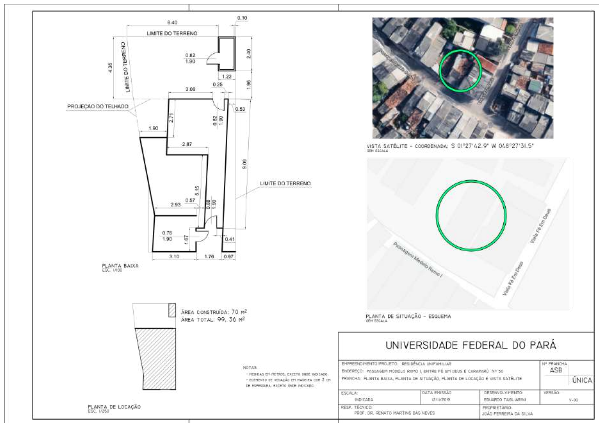
Planta Baixa I Residencial J.F.Silva, 2019.
