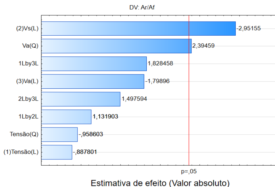
Figura 2. Gráfico de Pareto da resposta Ar/Af.
