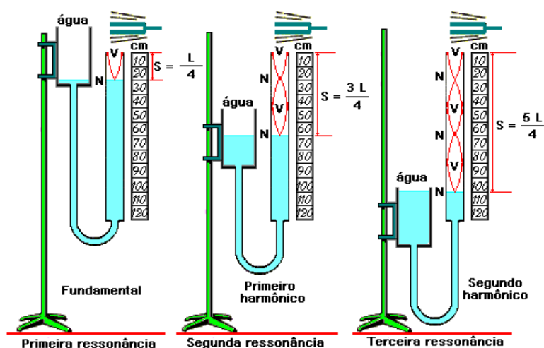
Figura 14: Harmônicos em tubos fechados
