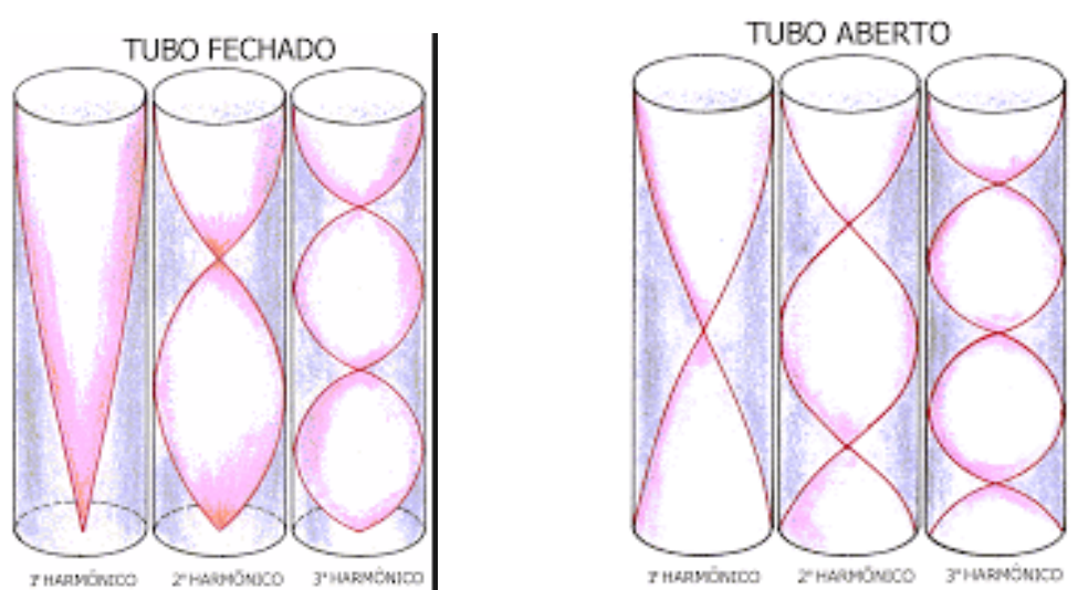
Figura 15: Tubo fechado – Nó e Ventre
